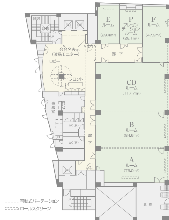
AP大阪梅田会場 平面図
